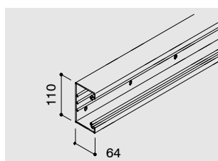
Csatornatest falra szerelhető kivitel Szállítási hossz: 2000 mm Fenékperforált
