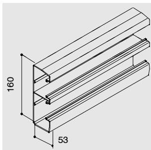
Csatornatest fedéllel falra szerelhető kivétel Szállítási hossz: 2000 mm Fenekperforált
