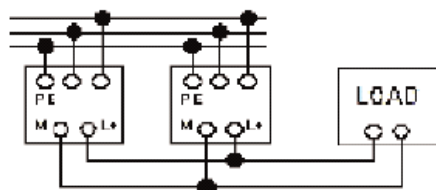
Egyfázisú készülékek párhuzamosítása
