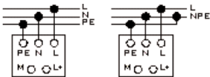
Bemeneti oldal bekötése
