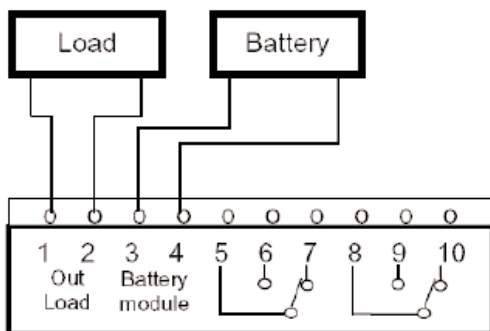
Fogyasztói és akkumulátor kimenetek bekötése, valamint a relés kimenetek (átjelzés) bekötési pontjai.
