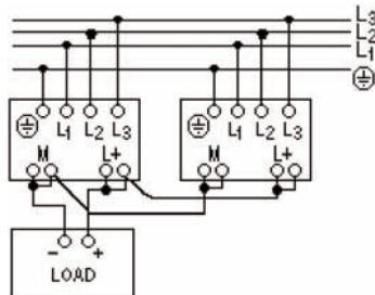
Háromfázisú készülékek párhuzamosítása
