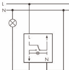
Nyomógomb, 1 pólusú (1 záróérintkező)
