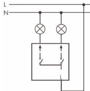
Csillárkapcsolás
