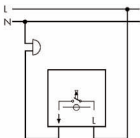
Nyomógomb, 1 pólusú (1 záróérintkező)
