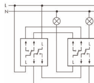
Váltókapcsolás
