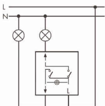
Csillárkapcsolás, jelzőfényel
