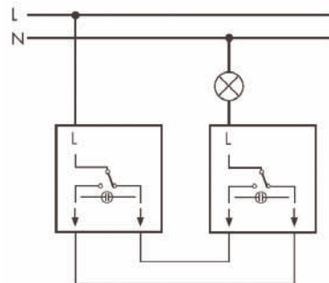
Váltókapcsolás
