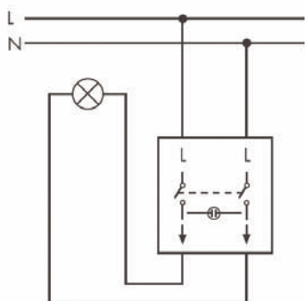
2 pólusú kontroll-kapcsolás
