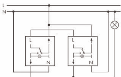
Csillárkapcsolás, jelzőfényel
